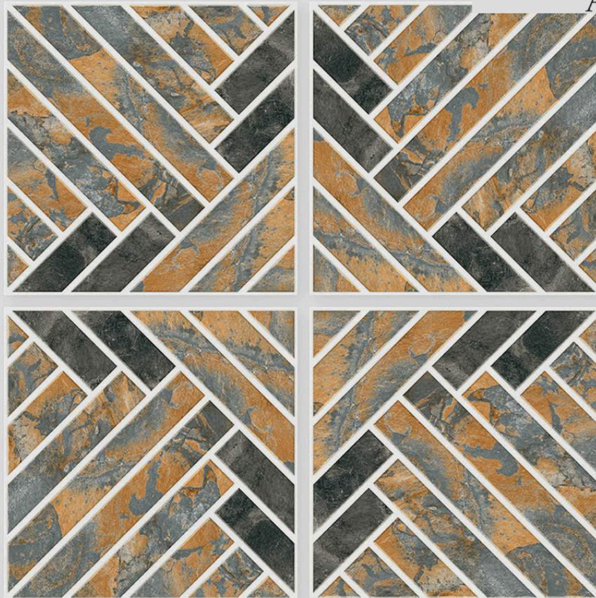
ONYX 07
